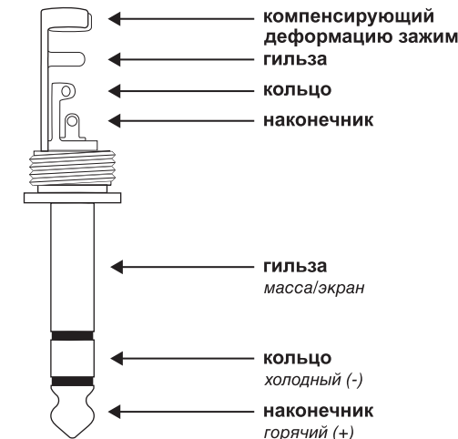
Рис. 3.2: 6,3-мм-монохраповый штекер
