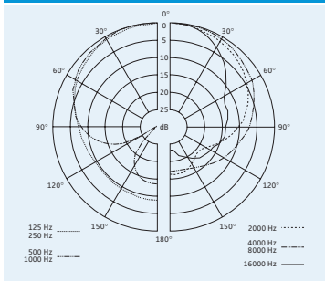
Полярная диаграмма MMD 845-1
