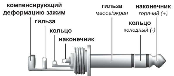
Рис. 4.5: 6,3-мм-стереоштекер
