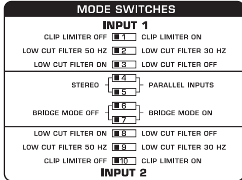
Рис. 2.3: DIP-переключатель EUROPOWER
