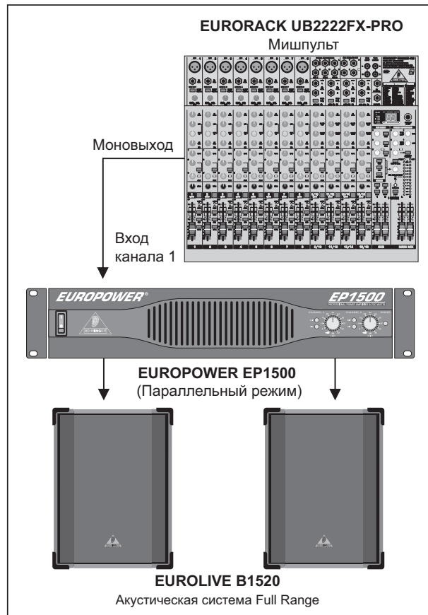
Рис. 3.3: Параллельный режим
