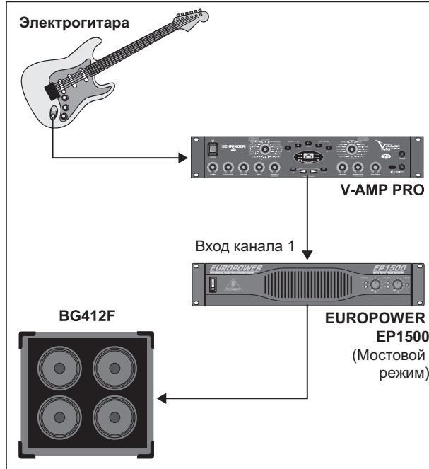
Рис. 3.5: Мостовой режим
