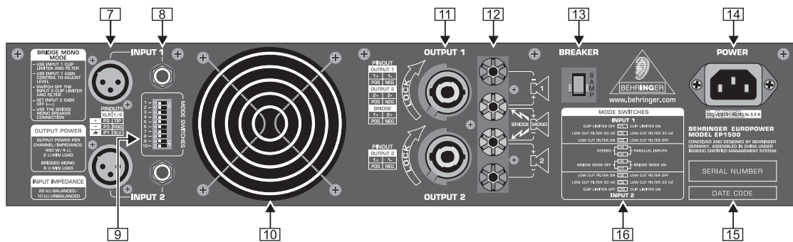
Рис. 2.2: Задняя панель, элементы управления и соединения
