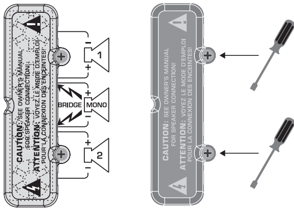
Рис. 4.2: Пластмассовая крышка, закрывающая соединительные клеммы
