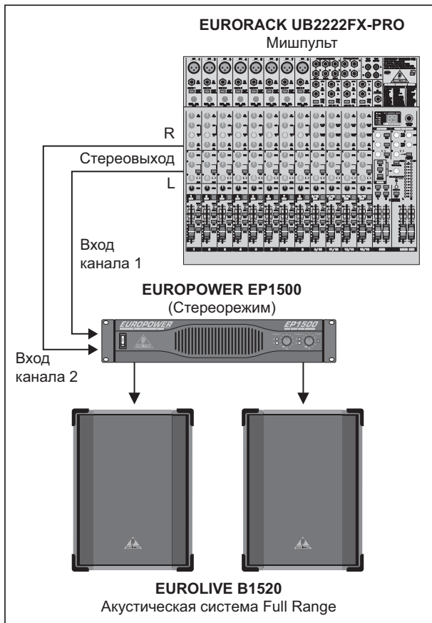
Рис. 3.1: Двухканальный режим
