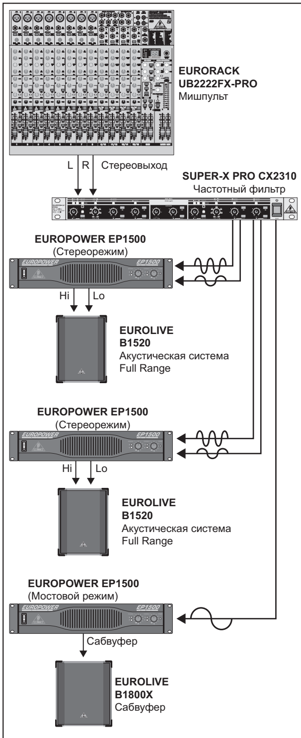
Рис. 3.7: Стереорежим Vi-Аmp с отдельным сабвуфером
