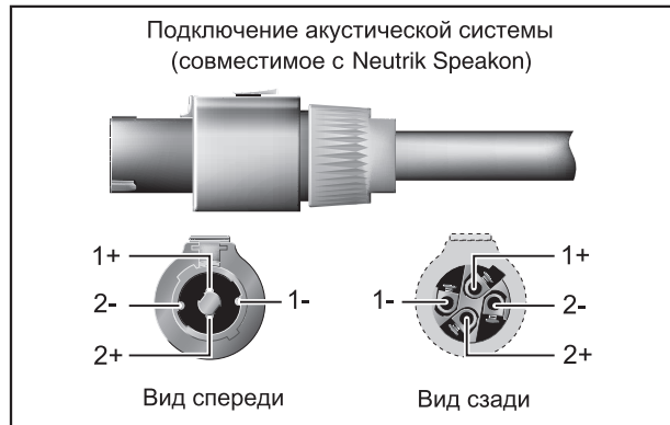
Рис. 4.1: Neutrik Speakon- совместимые разъемы
