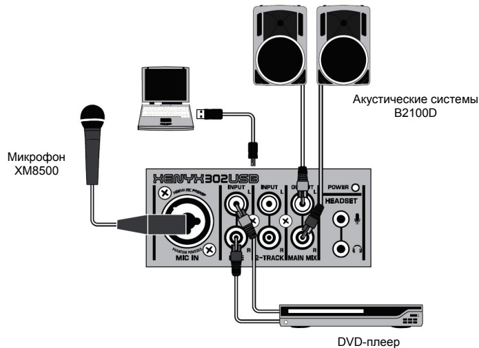
Система "Карaoke" с использованием DVD-плеера или компьютера
