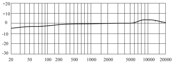
Частотный диапазон Meteor Mic
