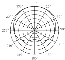
Диаграмма направленности Meteor Mic
